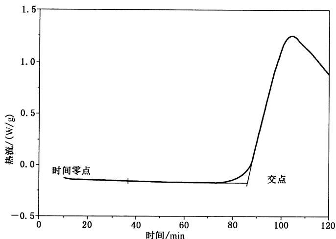
图 F.1 氧化诱导期的确定
